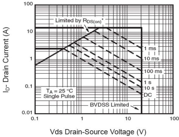
图 13 安全工作区域
