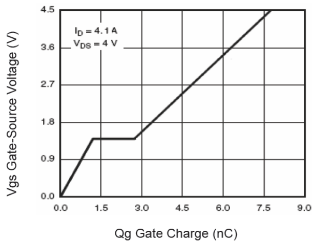
图 11 栅极电荷和电压关系
