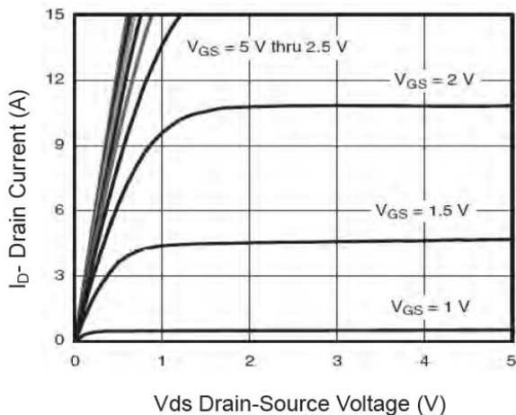
图 5 输出特性
