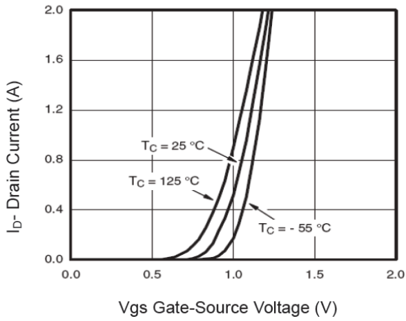
图 7 传输特性
