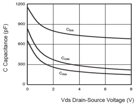
图 10 电容和 V_{DS} 关系
