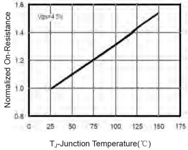
图 8 漏极和源极导通电阻
