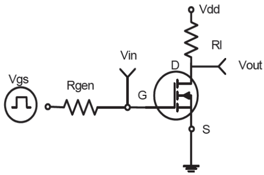
图一 开关测试电路
