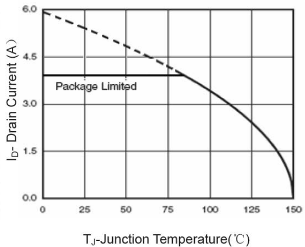
图四 漏极电流
