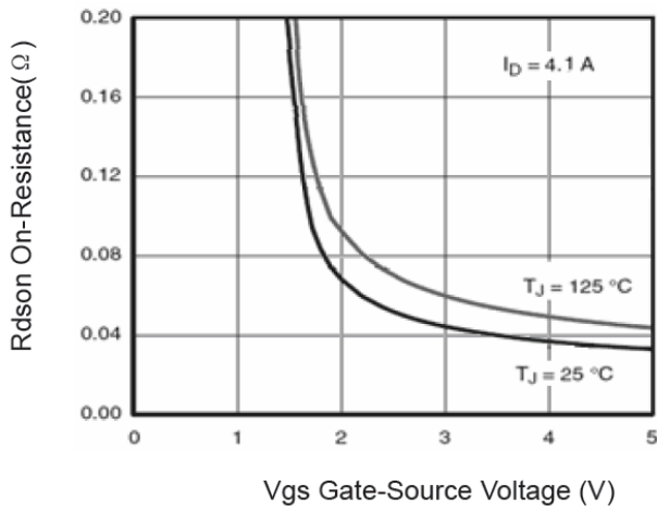
图 9 R_{DS(on)} 和 V_{GS} 关系
