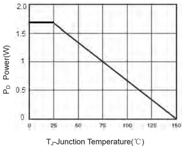
图三 功耗曲线
