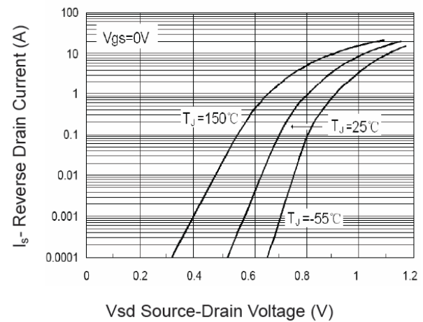
图 12 源极和漏极二级管导通特性
