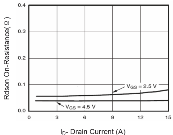
图 6 漏极和源极导通阻抗
