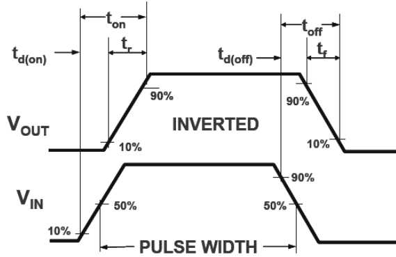
图二 开关波形
